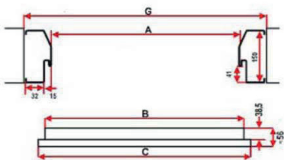
PROFIL „PD“, „PDT“ - vodorovný řez
