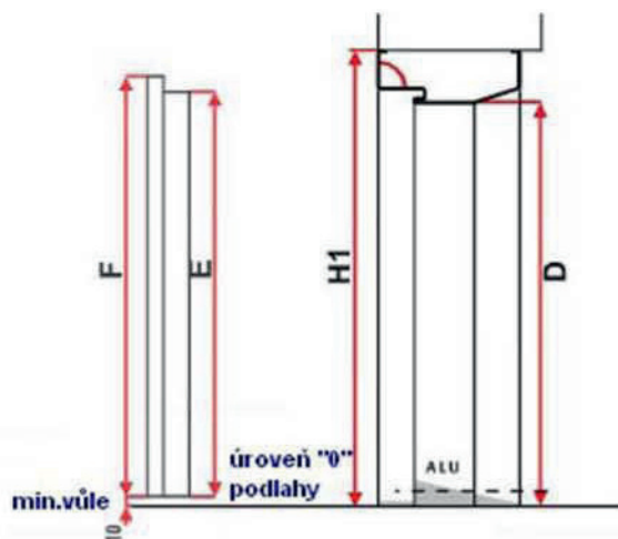
PROFIL „PD“, „PDT“ - svislý řez
